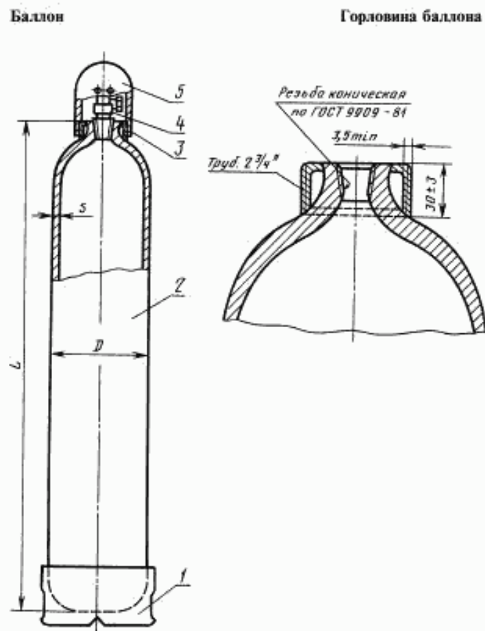
1 — опорный башмак; 2 — корпус баллона; 3 — кольцо горловины; 4 — вентиль; 5 — предохранительный колпак
